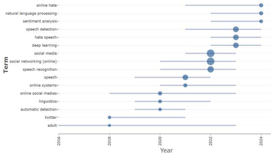
Fig. 15. Trend Topics
